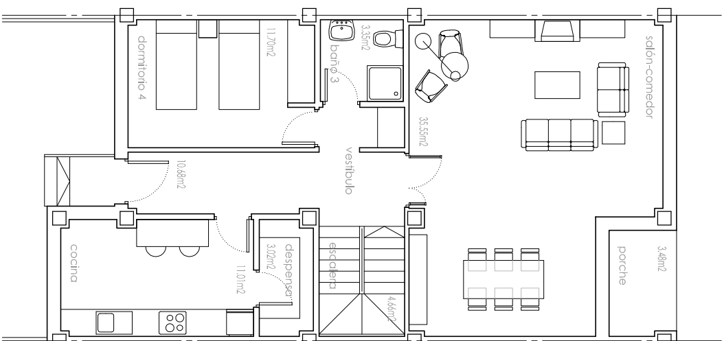
Planta Baja
