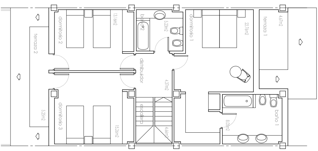
Planta Primera
