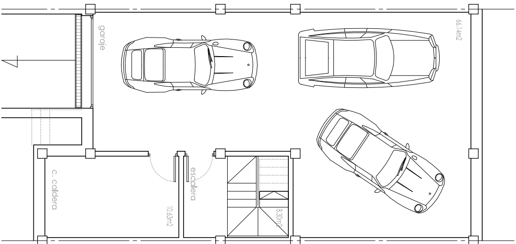
Planta Semisótano
